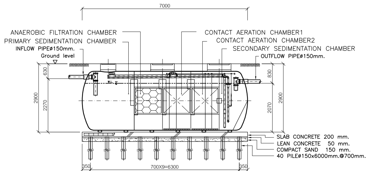
SECTION A-A
